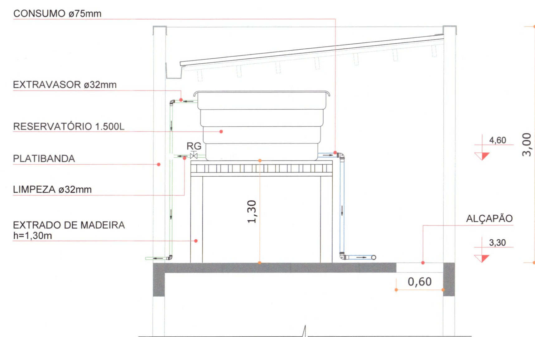
DETALHE EXTRAVASOR / LIMPEZA SEM ESCALA
