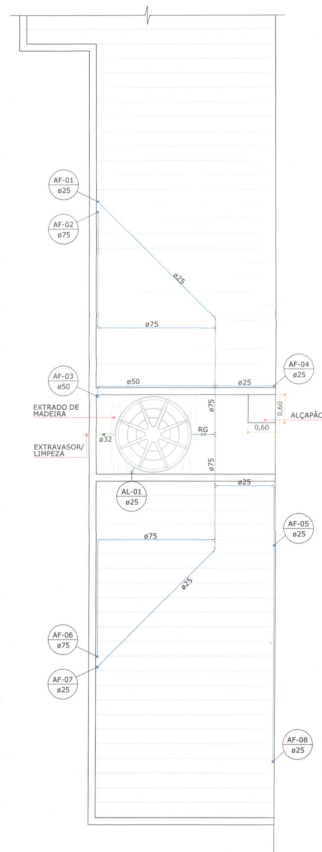
RESERVATÓRIO ESCALA | 1:125
