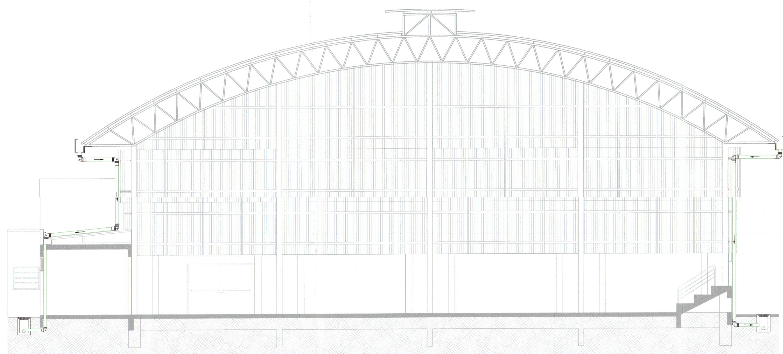
CORTE ESQUEMÁTICO ESCALA | 1:100
