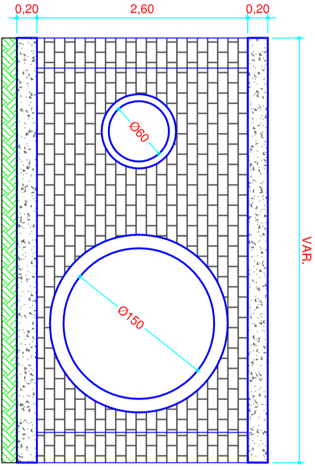
CORTE AA Obs.: dimensões em metros
