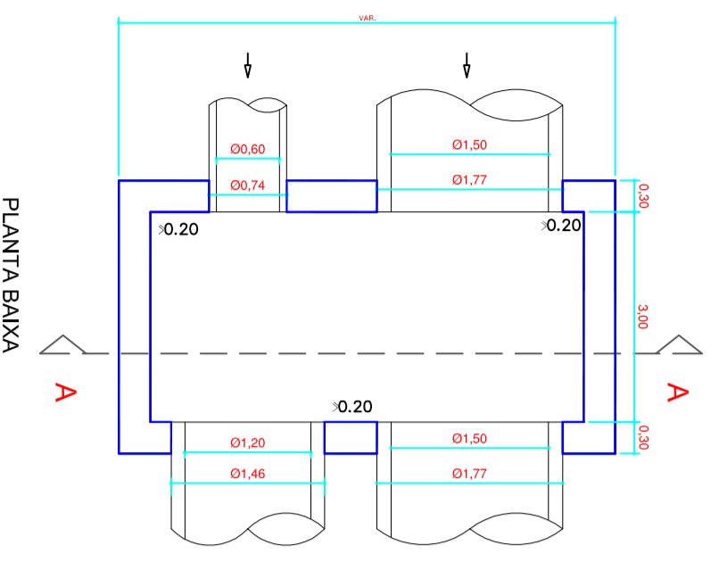
CAIXA DE INSPEÇÃO ESPECIAL 01
