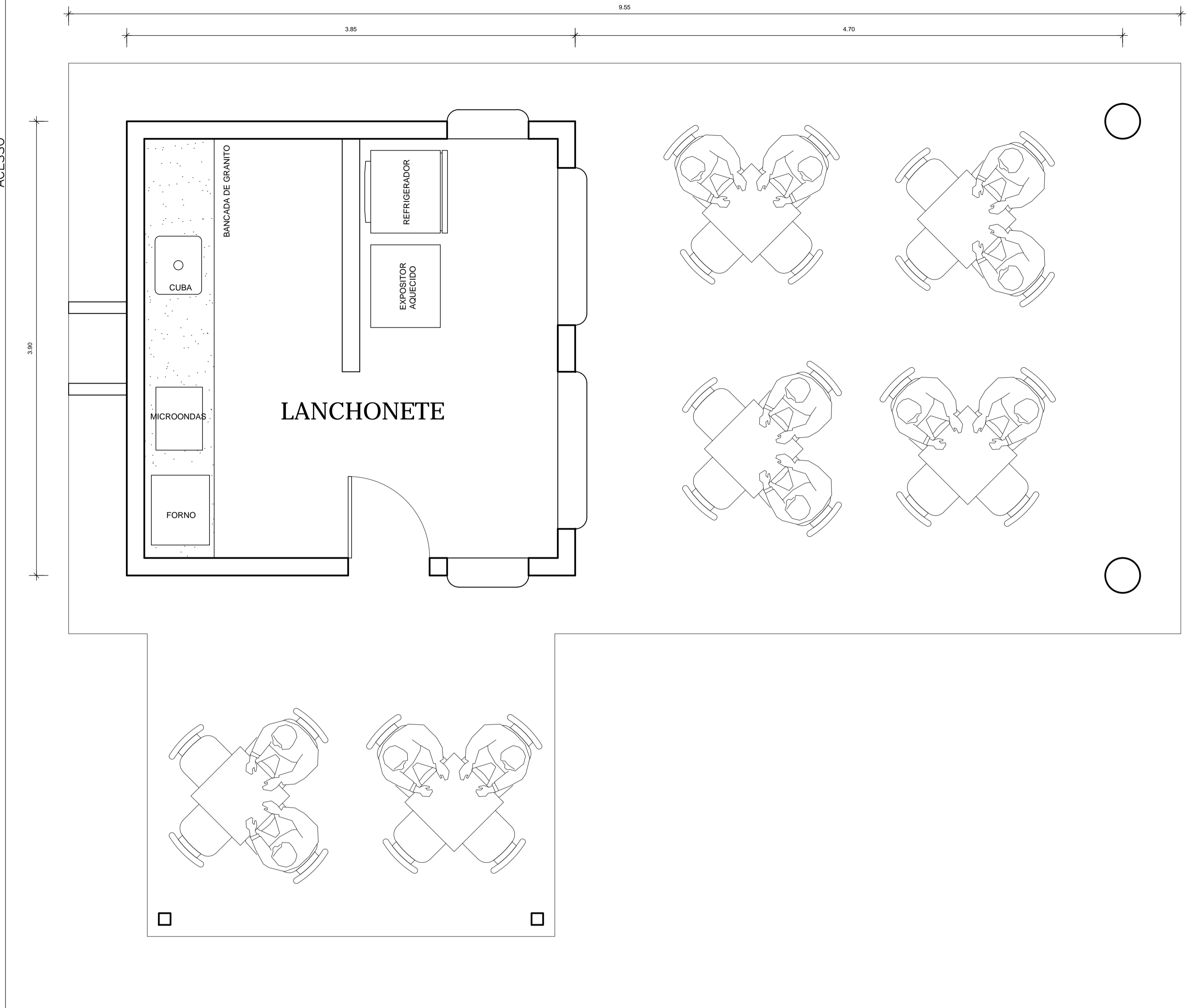
LAYOUT LANCHONETE Escala: 1:25
