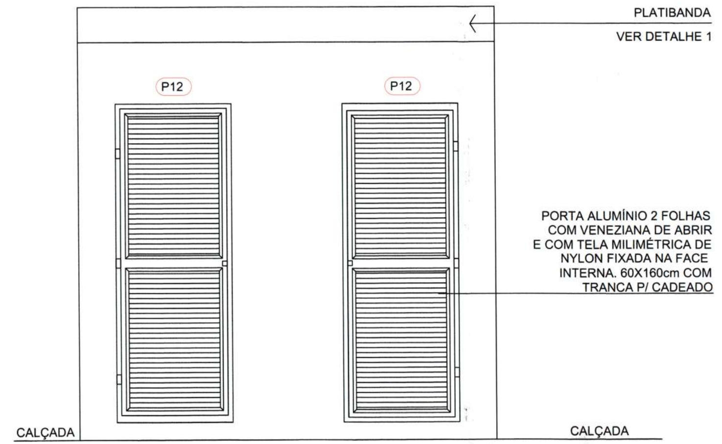
VISTA FRONTAL - DEP. LIXO SEM ESCALA
