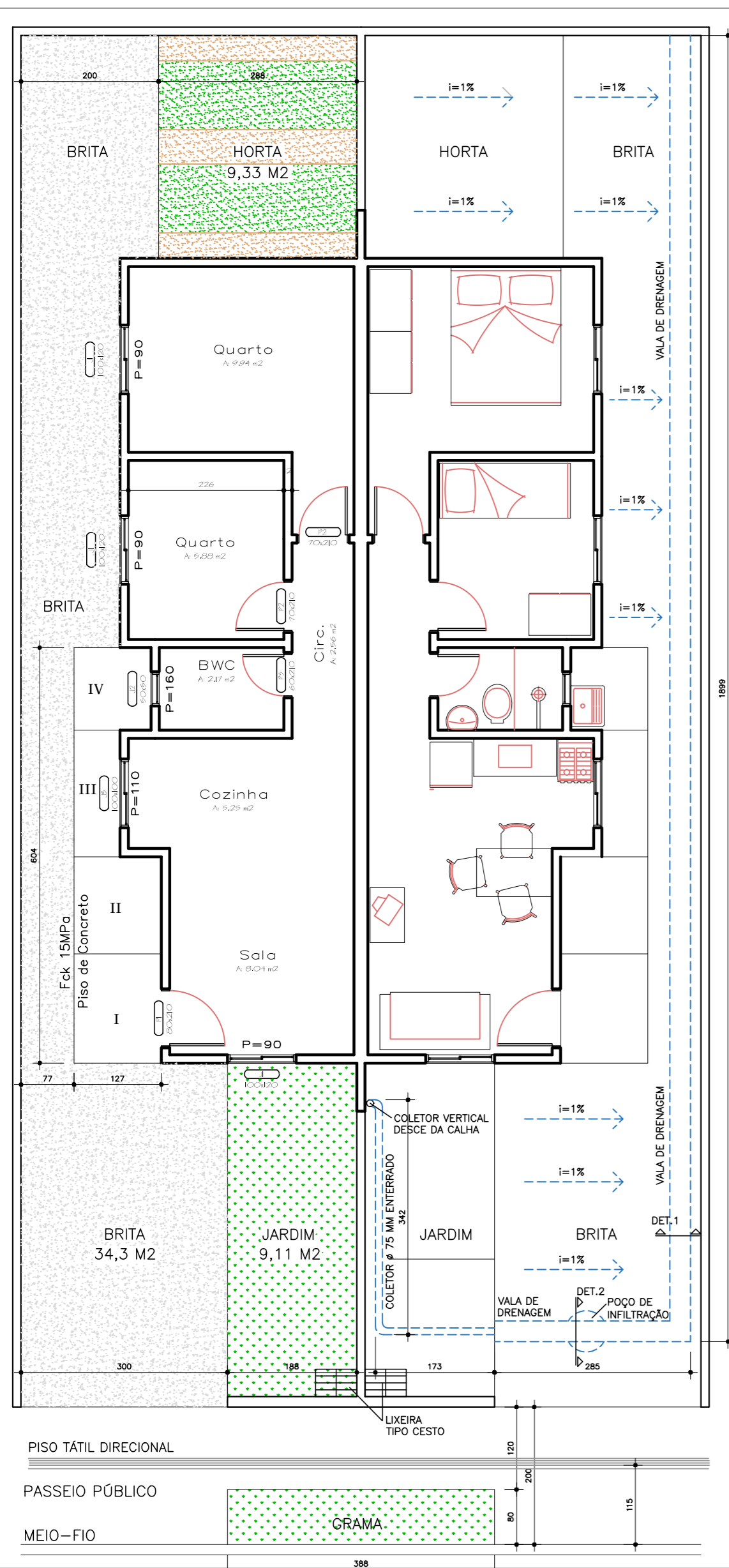
URBANÍSTICO ESC: 1/400
