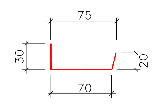
CORTE TRANSVERSAL DA CALHA METÁLICA TRAPEZOIDAL EXISTENTE - DIMENSÃO A SER MANTIDA NA INSTALAÇÃO DA NOVA CALHA EM ALUMÍNIO (CONFERIR MEDIDAS IN LOCO). S/ Escala
