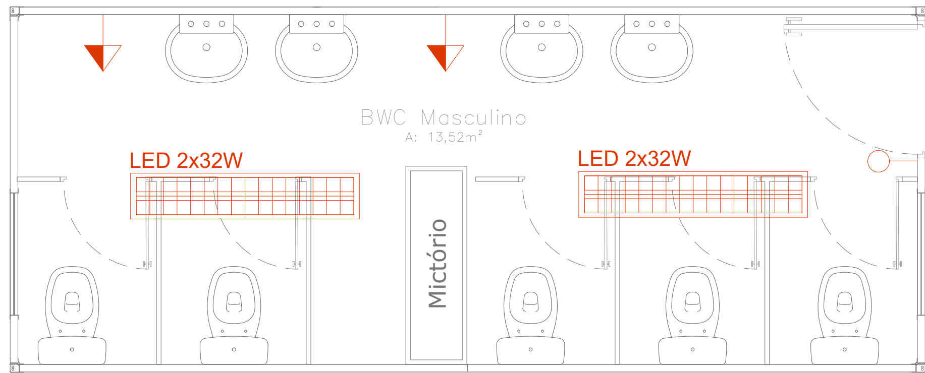
PLANTA BWC MASCULINO
