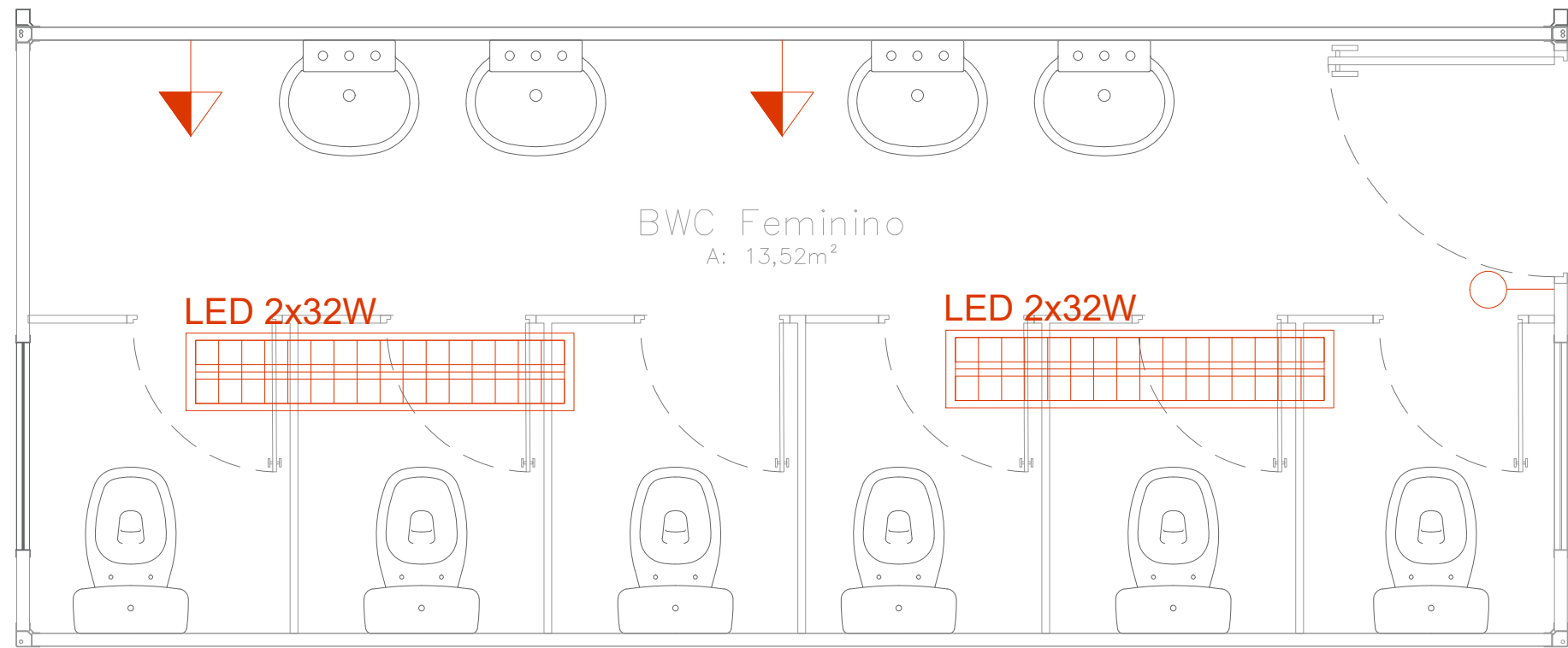
PLANTA BWC FEMININO
