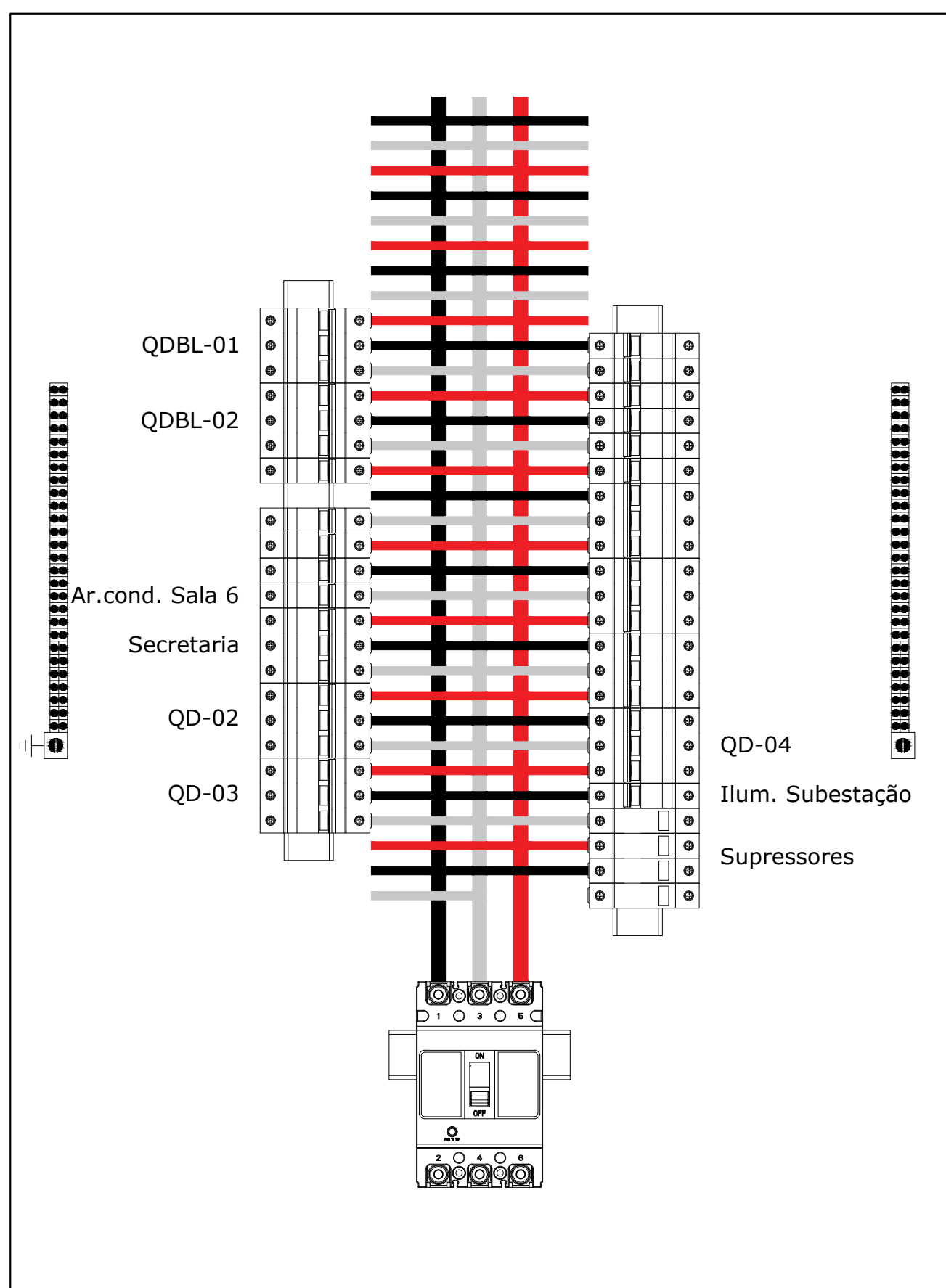
QGBT - EM SEM ESCALA
