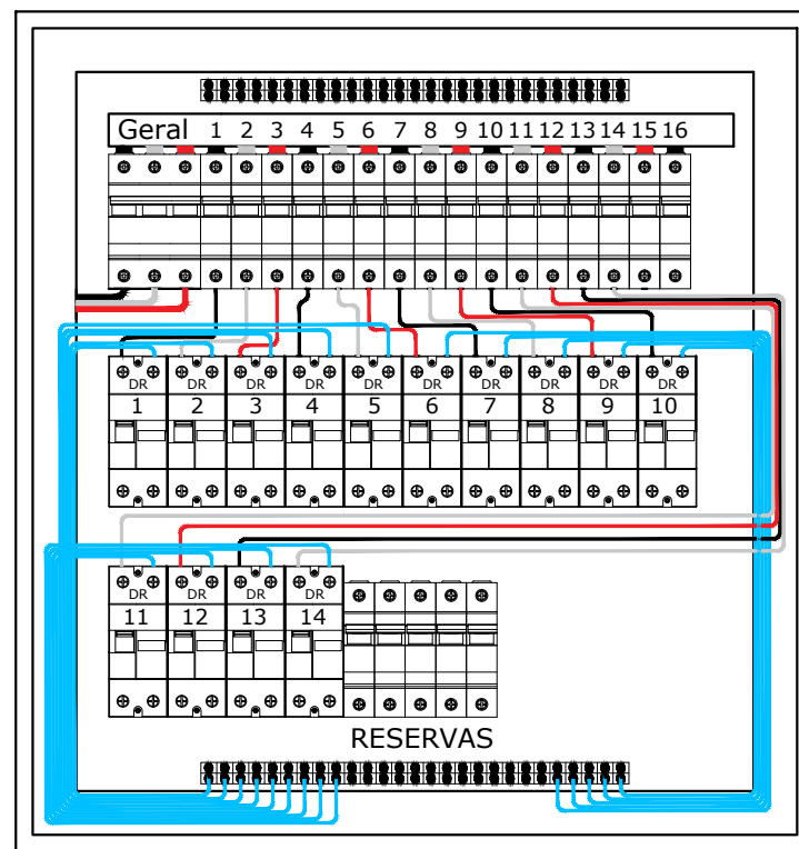
QDBL - 01 SEM ESCALA
