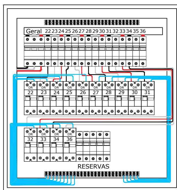
QDBL - 02 SEM ESCALA
