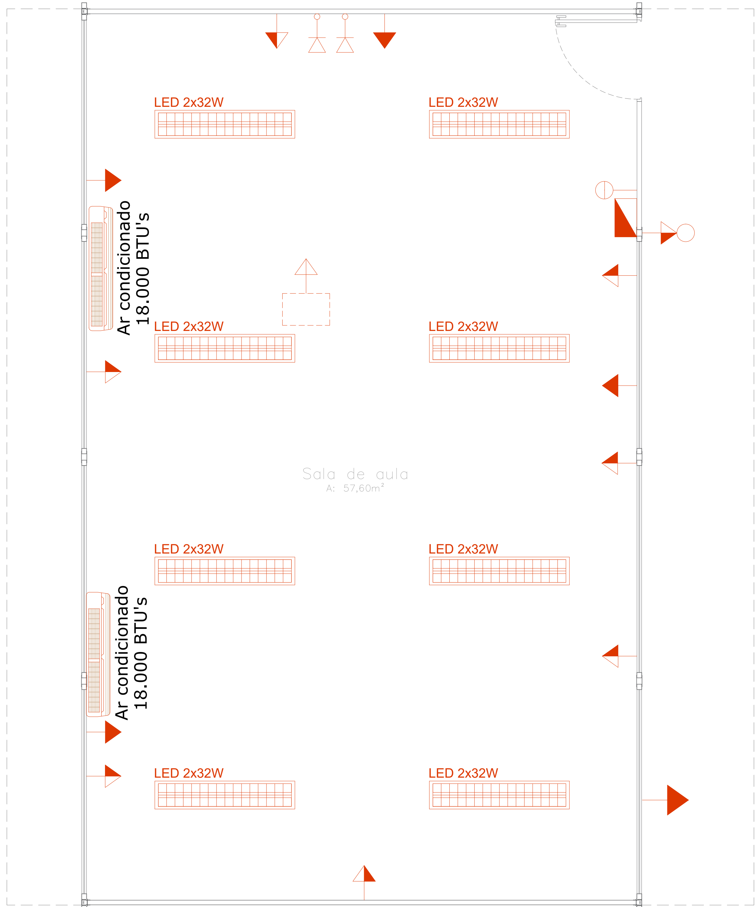
PLANTA SALA DE AULA
