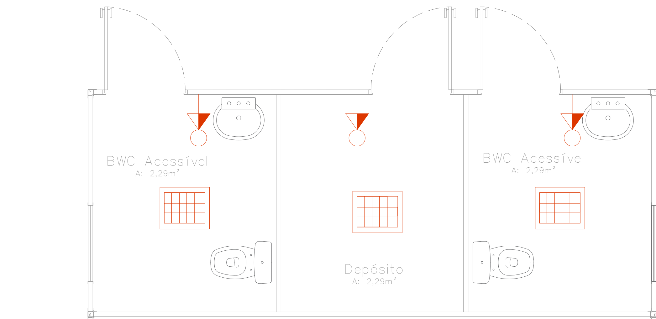
PLANTA BWC ACESSÍVEL E DEPÓSITO
