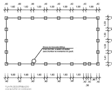
PLANTA DE DISTRIBUIÇÃO DO CONCRETO
