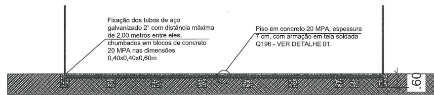
CORTE AA
