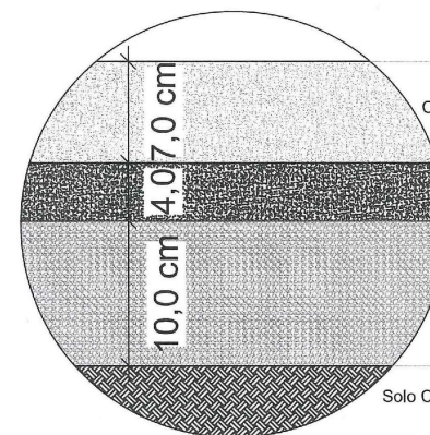
DETALHE 01
