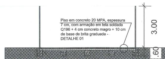
CORTE BB
