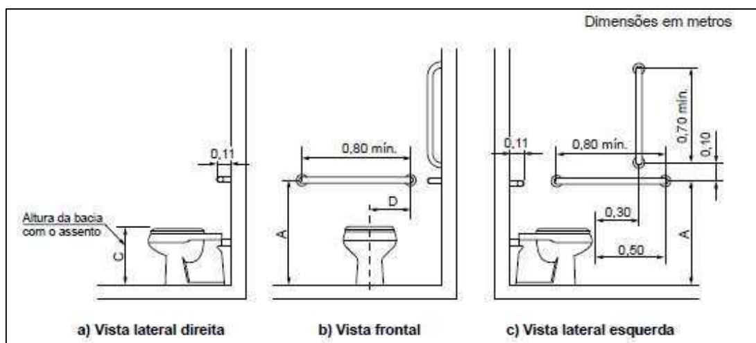
Figura 17 - Figura 11 – Barras de apoio para vaso sanitário
