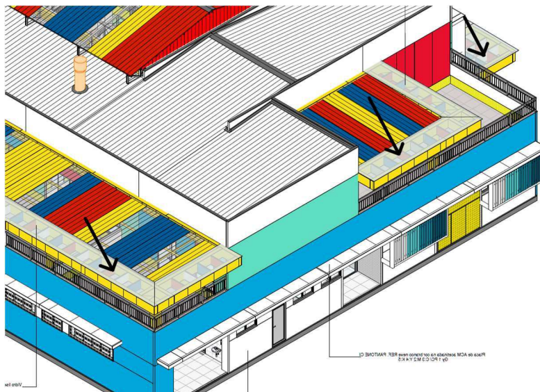
Figura 2 - Localização dos trechos que receberão vidro laminado
