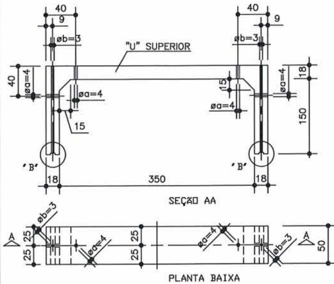
RELAÇÃO DO AÇO GAL350X150X50 - 'U' SUPERIOR
