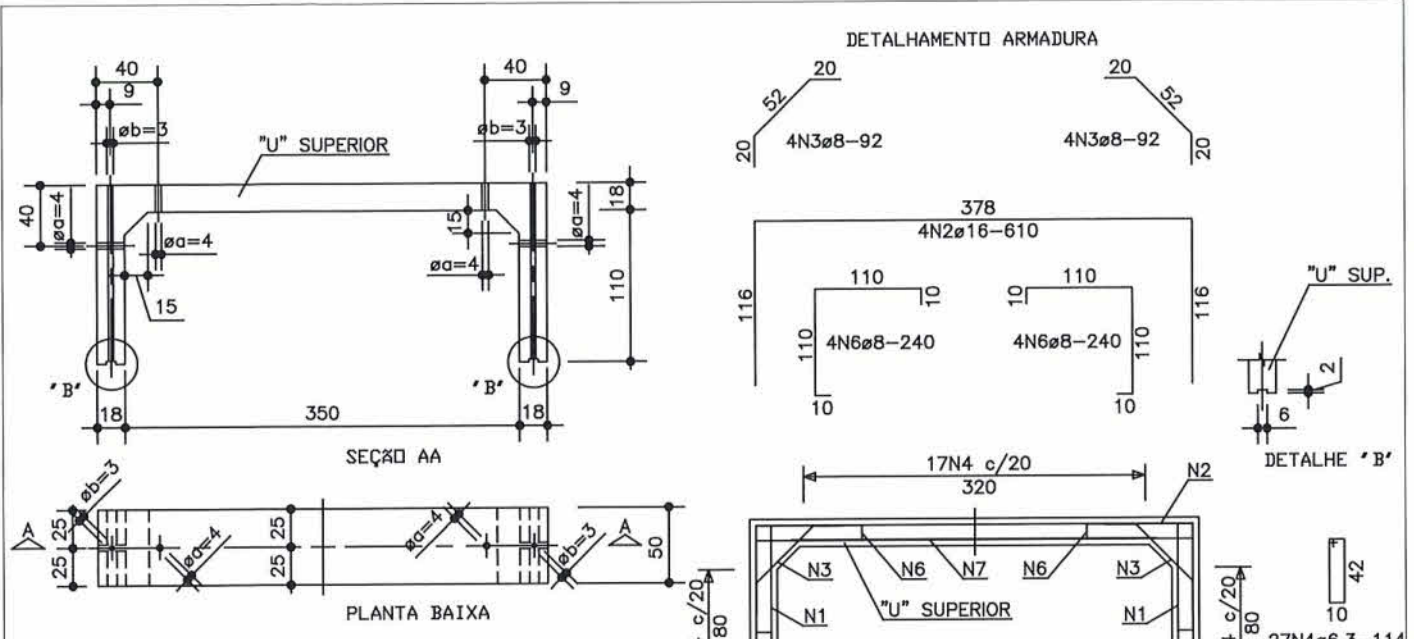
RELAÇÃO DO AÇO GAL350X110X50 - 'U' SUPERIOR
