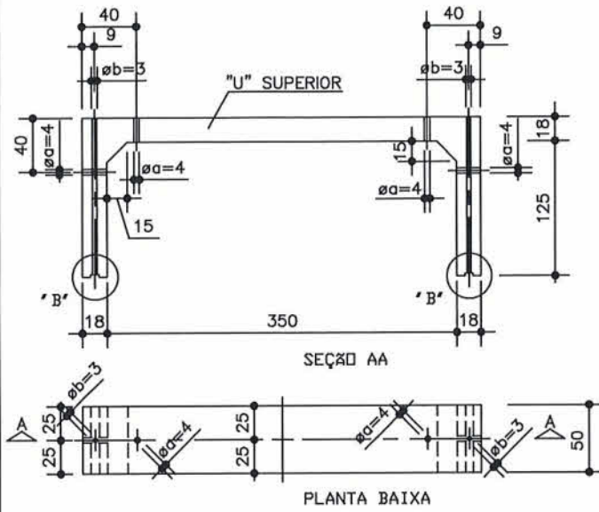
RELAÇÃO DO AÇO GAL350X125X50 - "U" SUPERIOR
