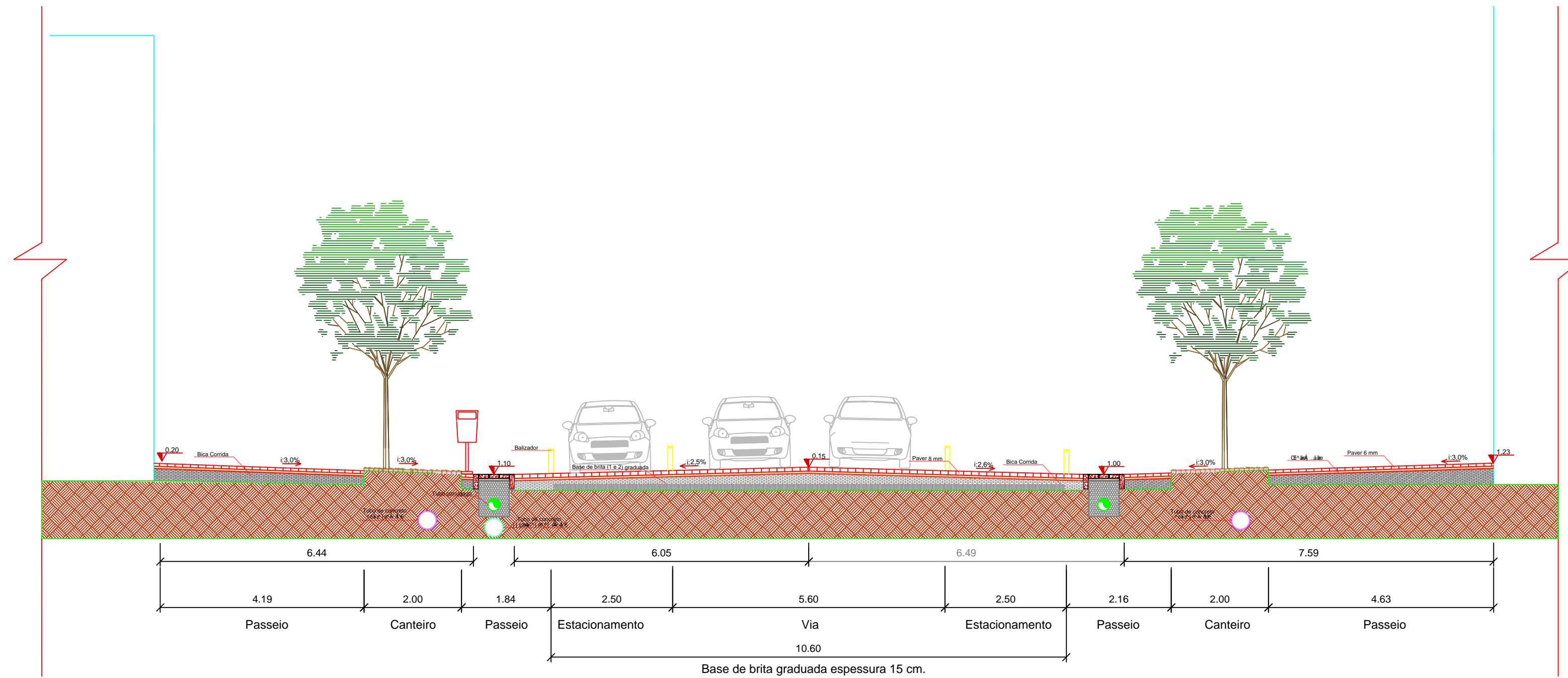
Corte AA' - Rua Dr. Noberto Bachmann Escala 1:75
