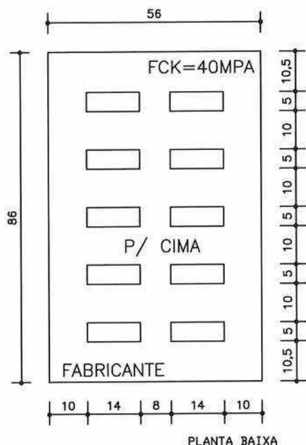
PLANTA BAIXA
