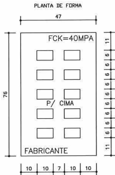
PLANTA BAIXA
