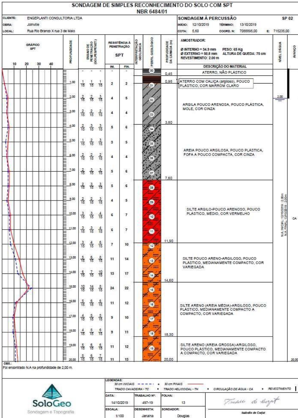
Sondagem SP02-2
