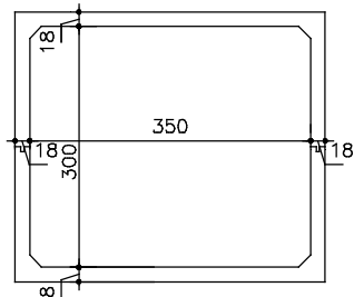
GALERIA PREMOLDADA EM CONCRETO ARMADO SEÇÃO 350x300
