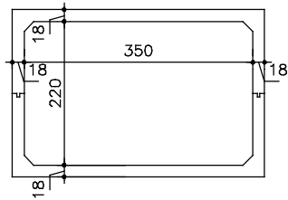
GALERIA PREMOLDADA EM CONCRETO ARMADO SEÇÃO 350x220
