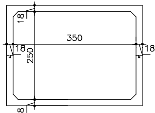
GALERIA PREMOLDADA EM CONCRETO ARMADO SEÇÃO 350x250
