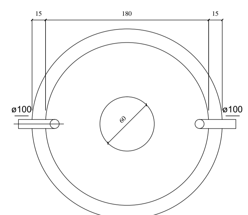
TANQUE SÉPTICO PLANTA BAIXA - ESC. 1:25
