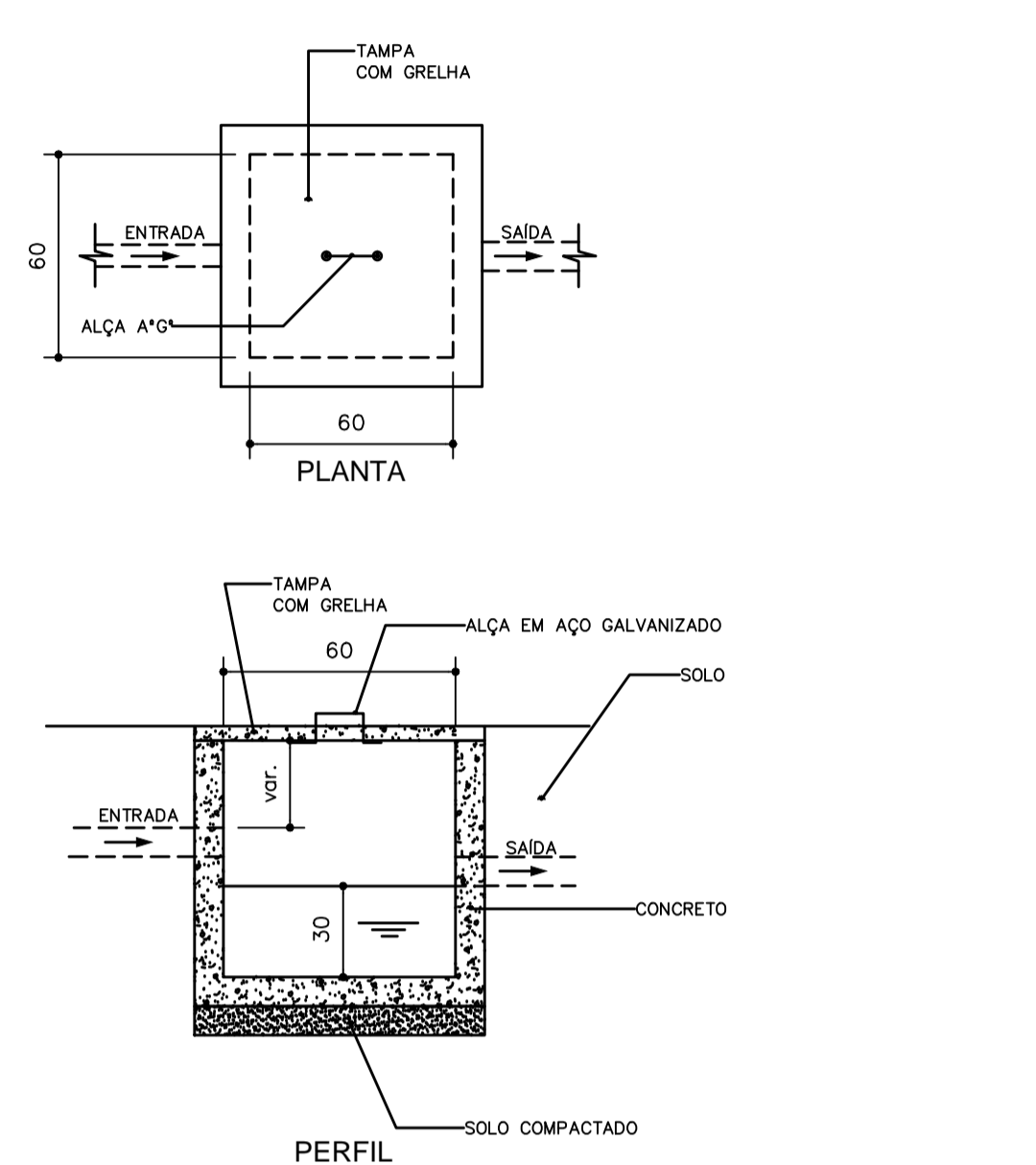
DETALHE CAIXA COLETORA DE AREIA ESC. 1/25
