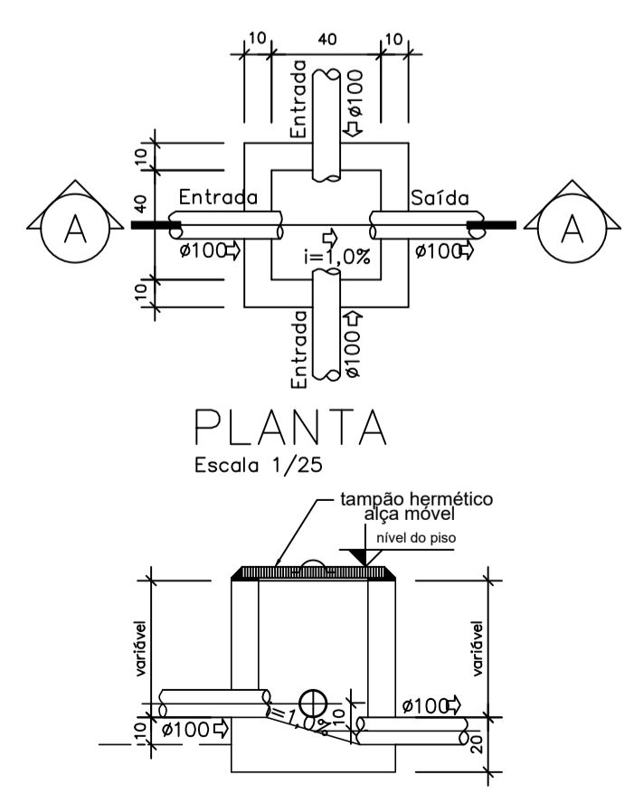
CAIXA DE INSPEÇÃO E PASSAGEM Escala 1/20
