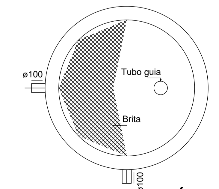
FILTRO ANAERÓBIO PLANTA BAIXA - ESC. 1:25
